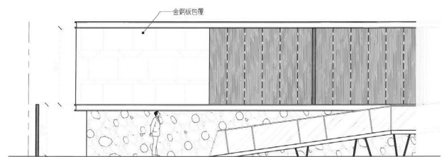
立面圖1
