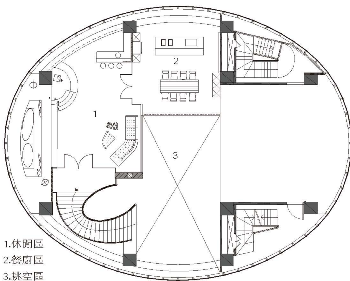
二層平面圖
