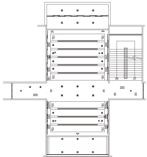
天花燈具圖
