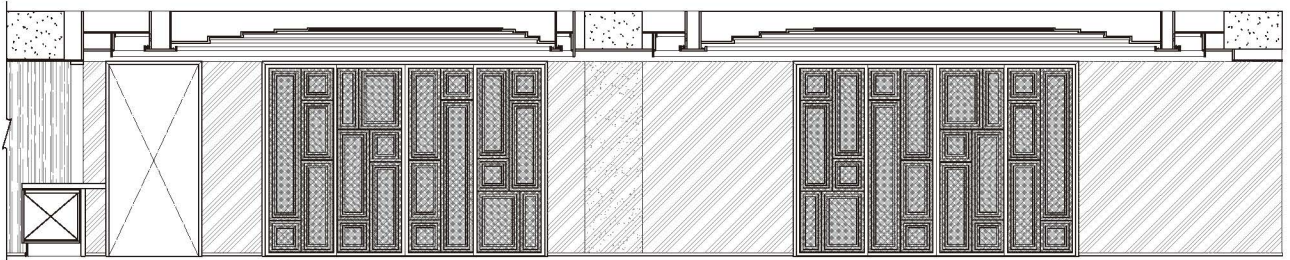
客廳餐廳立面圖
