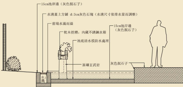
小瀑布盆器施工大樣圖
