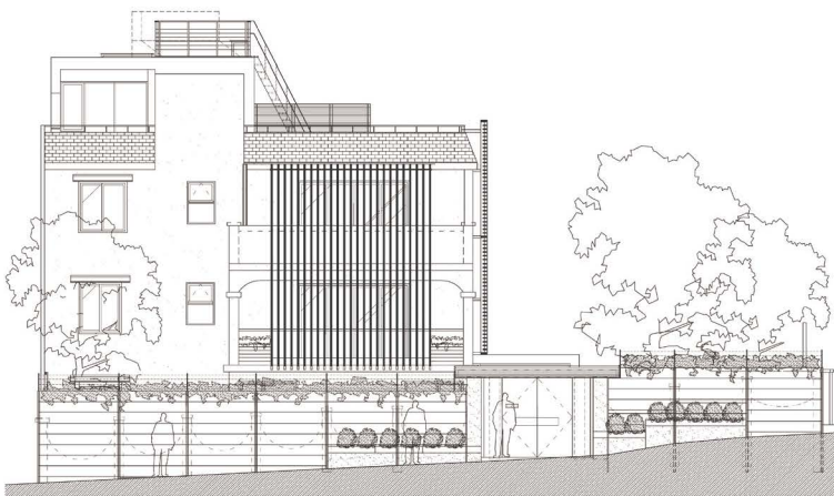
外觀立面圖
