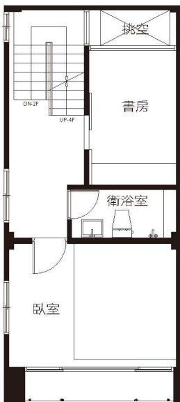
三樓平面圖
