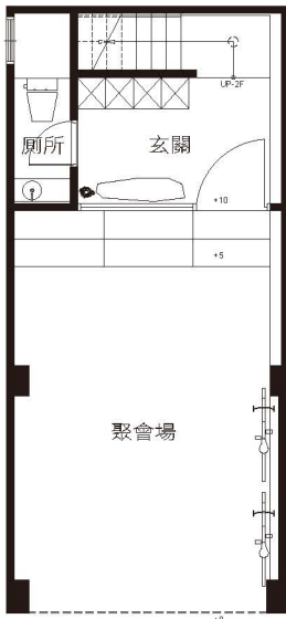
一樓平面圖
